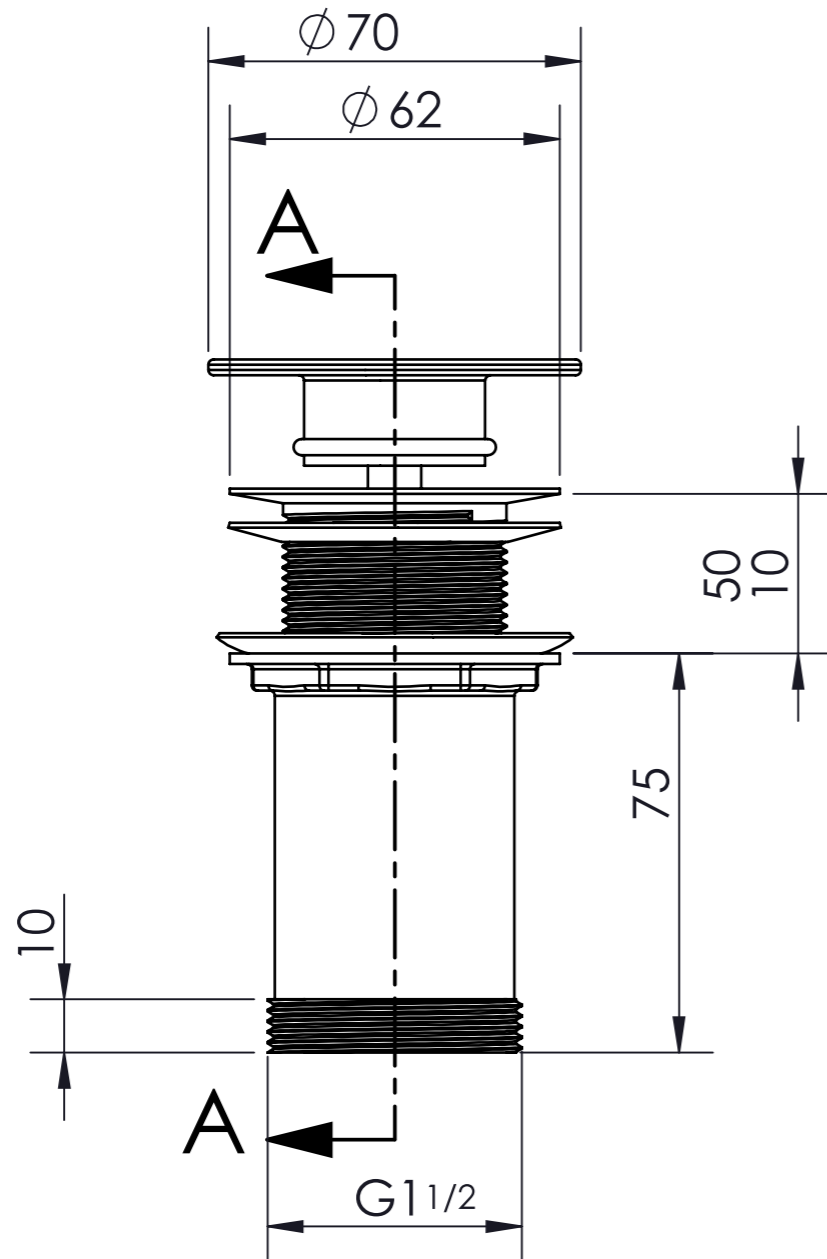
SECTION A-A
